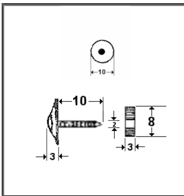
Σχέδια Κουμπιών Διαμέτρου 10 mm (Διαστάσεις σε mm)
